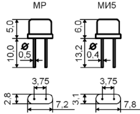
Рисунок 3 Резонатор РК466 Корпус МР
