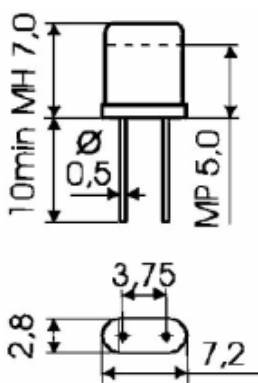
Рисунок 1 Резонатор РК542 Корпуса МН, МР
