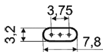
Рисунок 1 Корпуса МИ5
