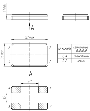
Рисунок 2 Резонатор РК536 Корпус СМД6
