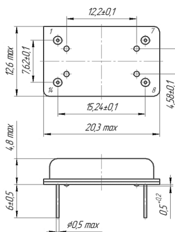
Рисунок 1 Генератор ГК261-П Корпус DIL-14
