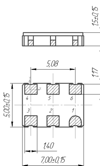
Рисунок 1 Генератор ГК406-П Корпус СМД7
