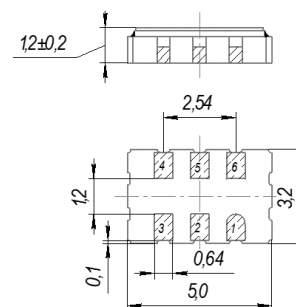
Рисунок 2 Генератор ГК304-УН-Л-01 Корпус СМД5
