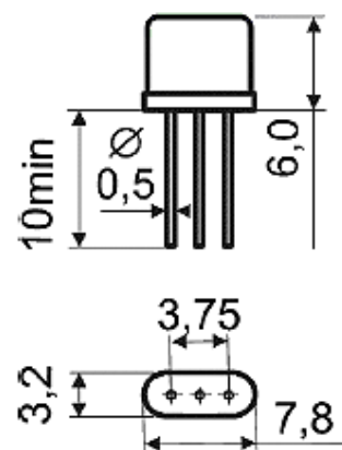
Рисунок 2 Корпус МИ5
