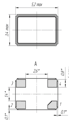
Рисунок 4 Резонатор РЛ561 Корпуса СМД5
