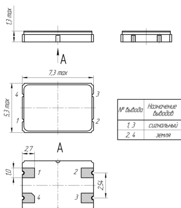
Рисунок 1 Резонатор РК536 Корпус СМД7
