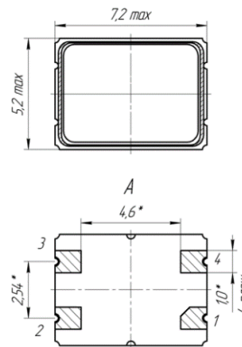
Рисунок 3 Резонатор РЛ561 Корпуса СМД7
