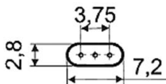
Рисунок 1 Корпуса МР
