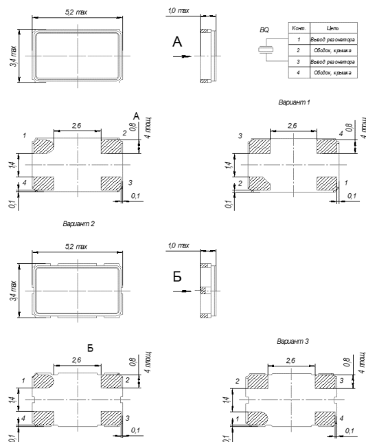
Рисунок 3 Резонатор РК560 Корпуса СМД5
