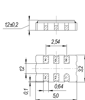
Рисунок 2 Генератор ГК303-УН-П-01 Корпус СМД5
