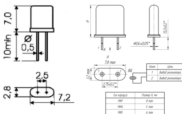
Рисунок 2 Резонатор РК543 Корпус ММ
