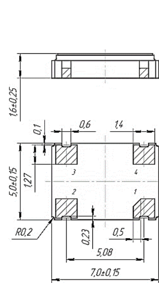
Рисунок 2 Генератор ГК261-П-П-01, ГК261-П-П-04 Корпус СМД7
