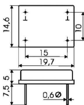
Общий вид, габаритные, установочные и присоединительные размеры фильтров ФП2П4-562, ФП2П4-563, ФП2П4-564, ФП2П4-564-01
