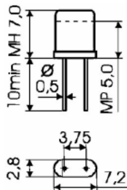
Рисунок 1 Резонатор РК419 Корпус МН и МР
