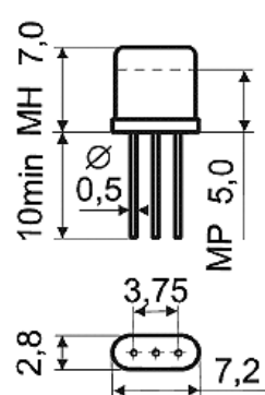
Рисунок 1 Корпуса МН и МР
