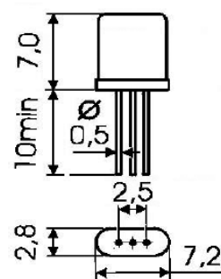
Рисунок 2 Корпус ММ
