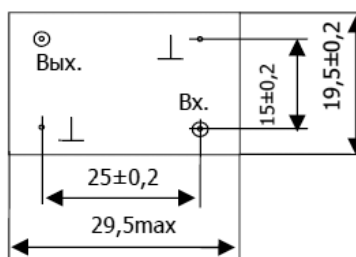
Рисунок 1 Фильтры ФП2П4-593, ФП2П4-593-01 Корпус 29,5x19,5x5 мм
