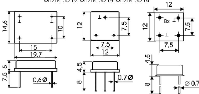
Рисунок 1 Корпуса «Терек»
