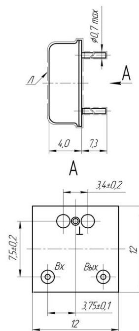
Рисунок 2 Фильтры ФП2П4-683-01 Корпус «Посол»
