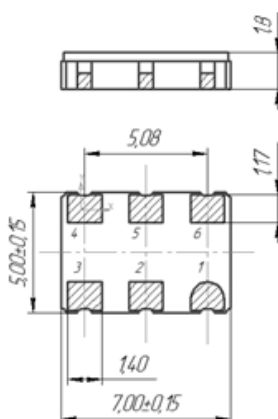
Рисунок 1 Генератор ГК304-УН-П Корпус СМД7
