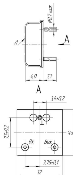
Рисунок 3 Фильтры ФПЗП4-783-04 Корпус «Посол»
