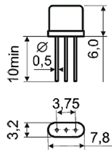
Рисунок 2 Корпус МИ5
