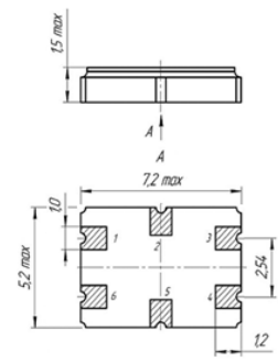
Рисунок 3 Корпус СМД7
