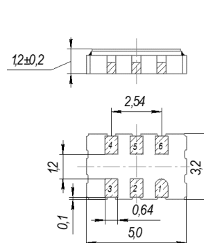
Рисунок 2 Генератор ГК304-УН-П-01 Корпус СМД5
