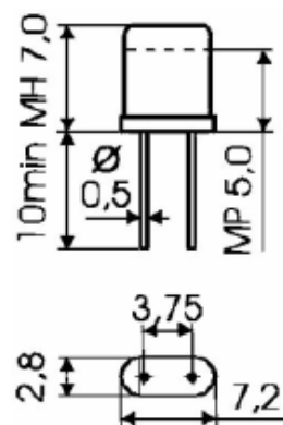
Рисунок 1 Резонатор РК419Т Корпус МН и МР
