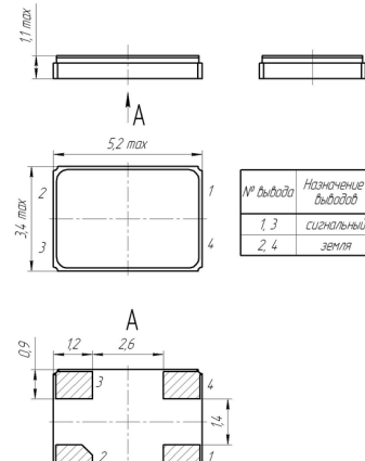
Рисунок 3 Резонатор РК536 Корпус СМД5
